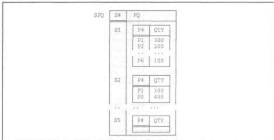
Рис. 12.17. Переменная отношения SPQ с атрибутом, содержащим в качестве значений другое отношение
