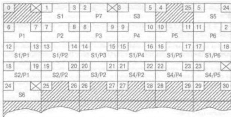
Рис. Г.4. Пересмотренный вариант рис. Г.3, на котором показаны указатели "следующей страницы" (в верхнем правом углу каждой страницы)
