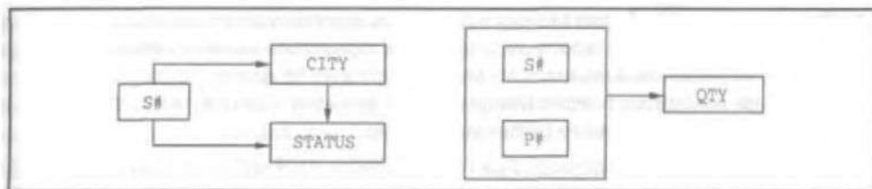
Рис. 12.7. Функциональные зависимости в переменных отношения SECOND и SP
