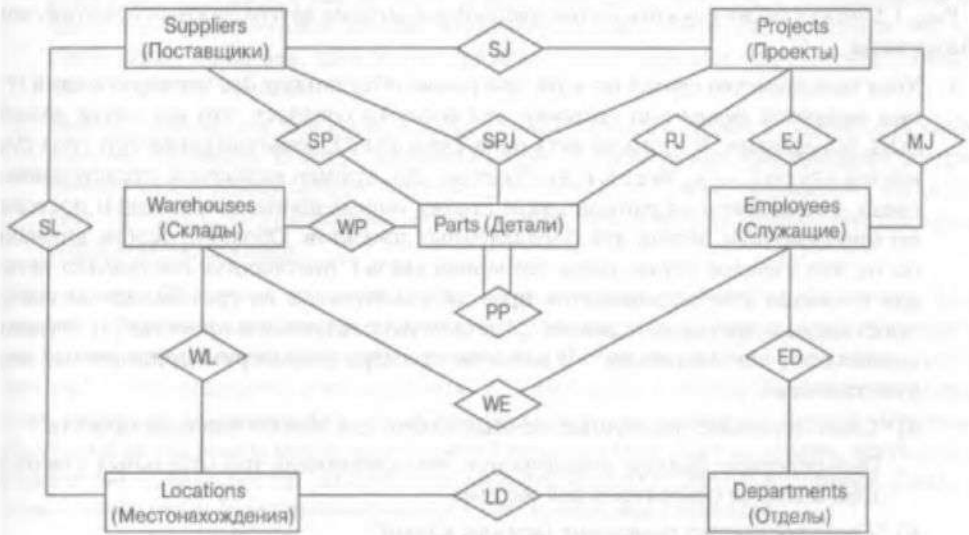
Рис. 1.5. Пример диаграммы "сущность-связь" (ER-диаграммы) для базы данных компании KnowWare, Inc.
