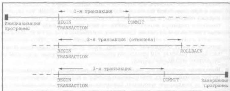
Рис. 15.2. Диаграмма, на которой процесс выполнения программы показан как ряд транзакций
