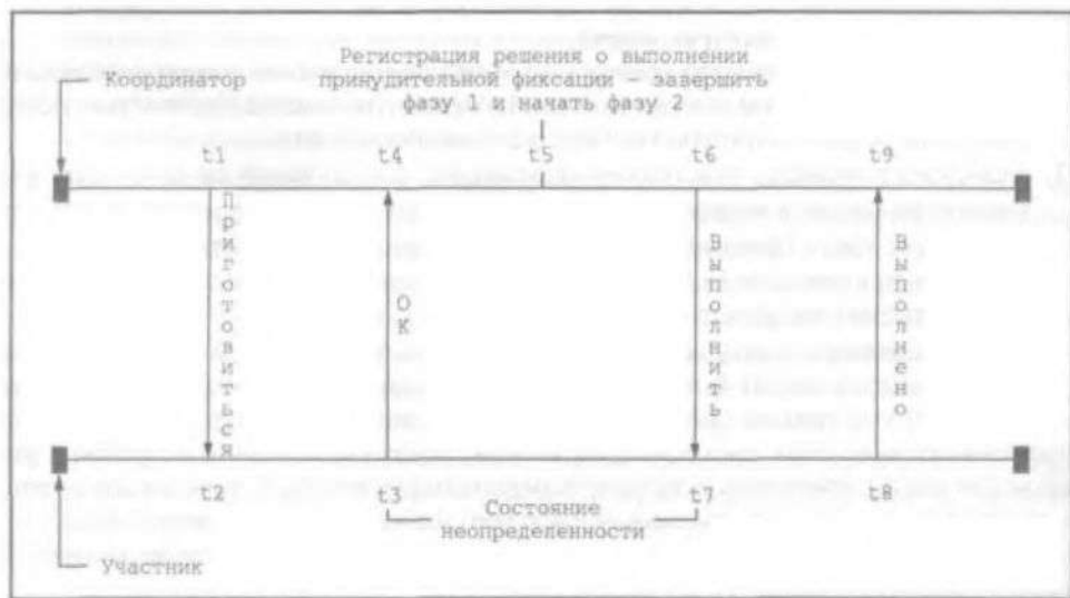
Рис. 21.4. Двухфазная фиксация транзакции
