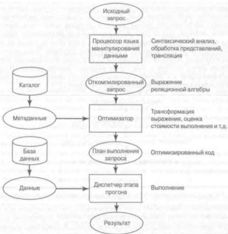
Рис. 18.1. Общая схема процесса оптимизации запроса
