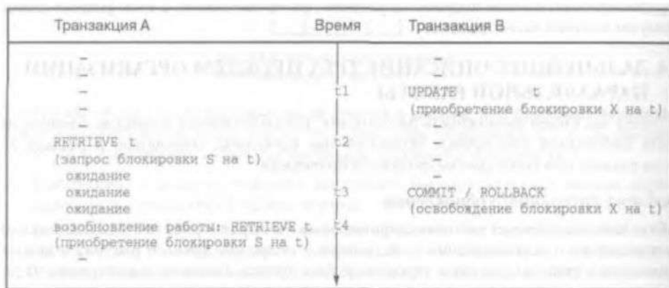
Рис. 16.7. Пример того, что для транзакции А исключена возможность считывать незафиксированное изменение в момент времени t_2
