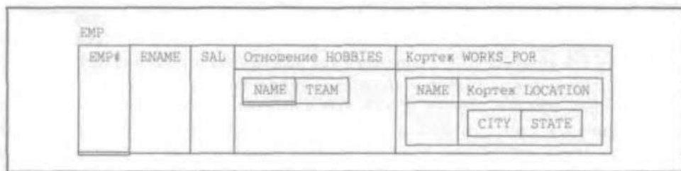
Рис. 26.2. Атрибуты, содержащие множества кортежей (указателей на кортежи), — нерекомендуемый вариант
