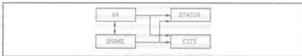
Рис. 12.12. Диаграмма функциональных зависимостей в переменной отношения S для случая, когда множество атрибутов {SNAME} является ее потенциальным ключом (и зависимость CITY \rightarrow STATUS не выполняется)
