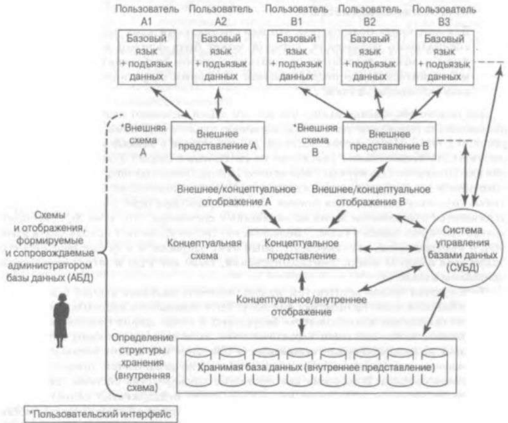
Рис. 2.3. Подробная схема архитектуры системы баз данных
